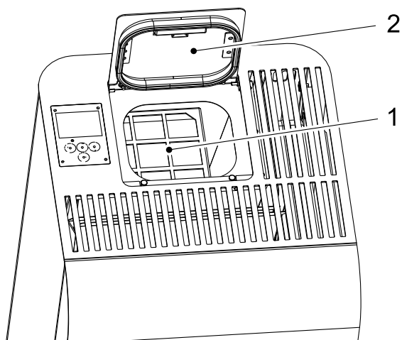
Obrázek 4: Zásobník na pelety
