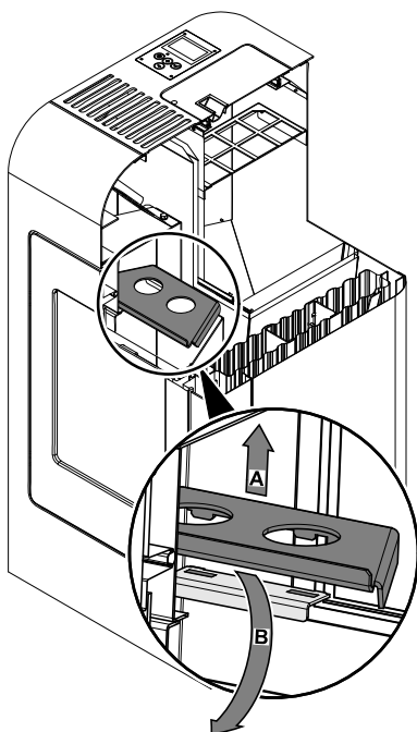
Obrázek 2: Demontáž desky přesměrování tahu
