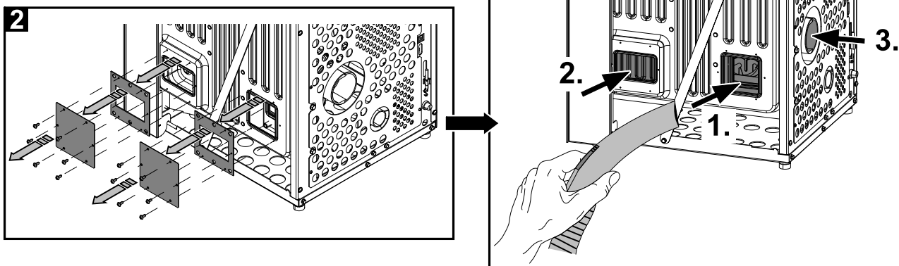
Obrázek 3: Demontáž boční stěny
