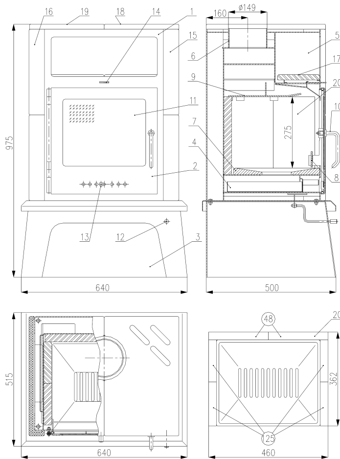
Šamotová vyzdívka
